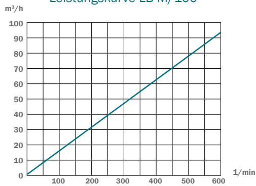
Leistungskurve LB-M/100
