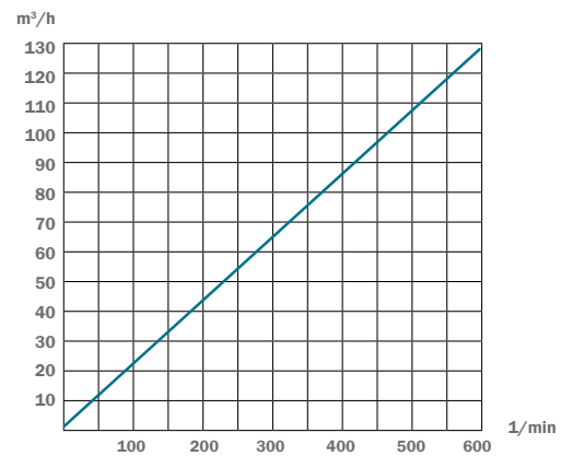
Leistungskurve LB-M/125
