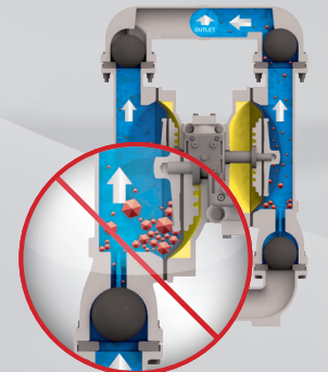
Top Discharge
